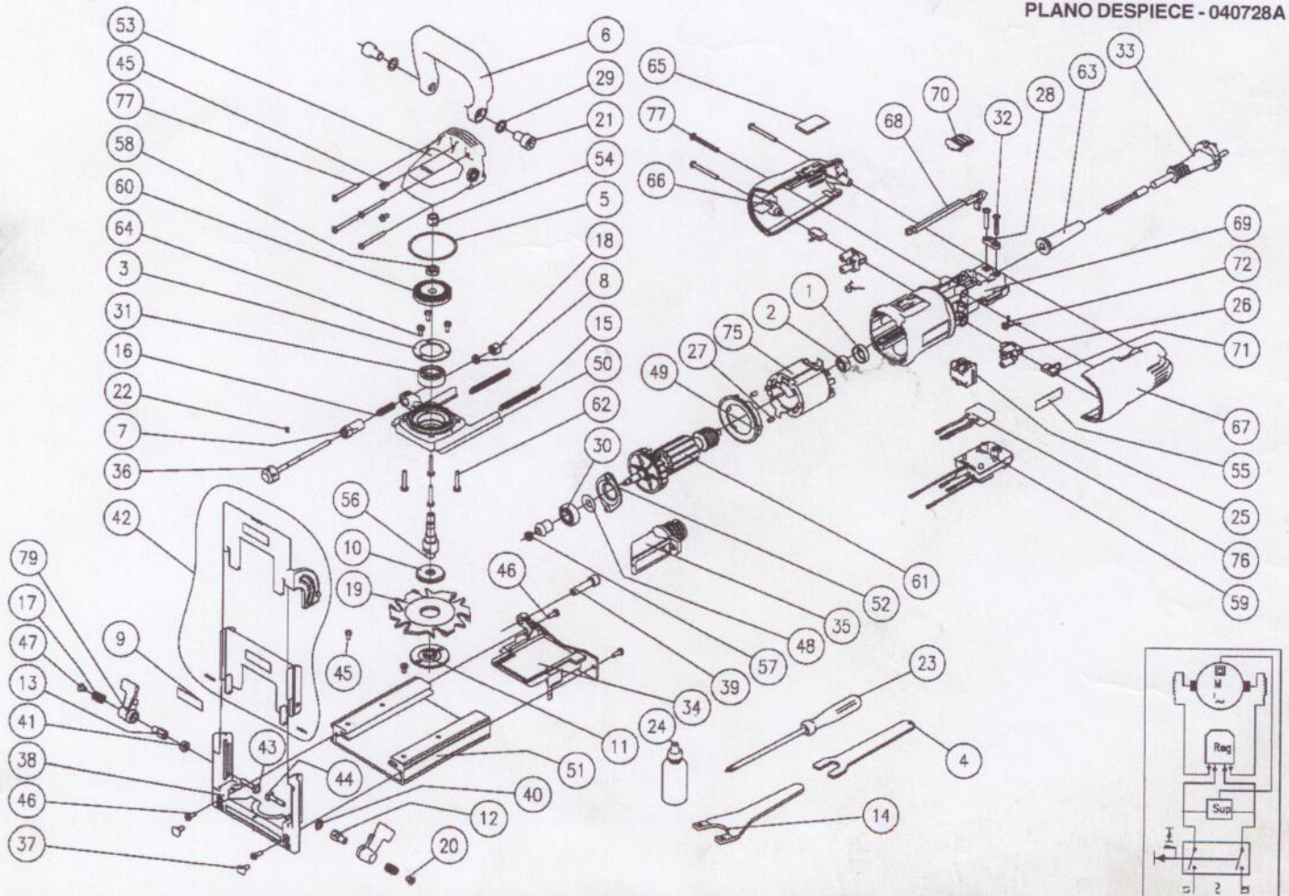
PLANO DESPIECE - 040728A
